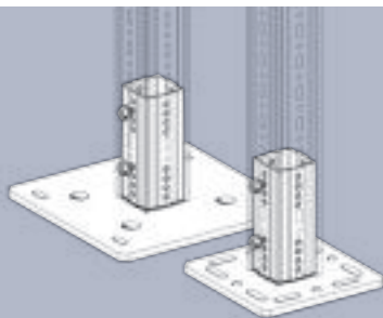
Držiak WBD F 80 Držiak WBD F 100 Držiak WBD F 100/160
